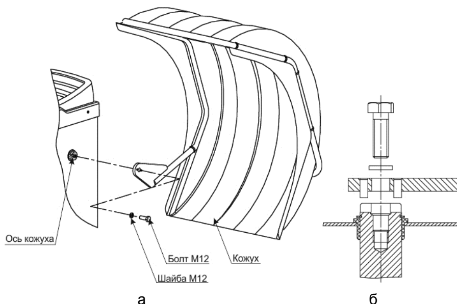
Рисунок 4.3 – Установка кожуха
